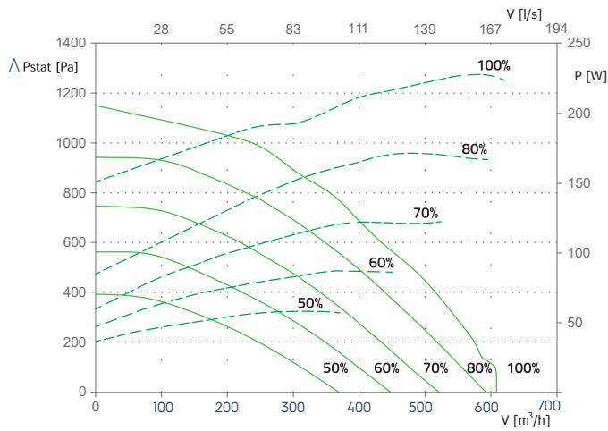
Toevoerlucht
