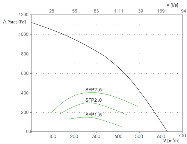
Specifiek ventilatorvermogen (SFP)
