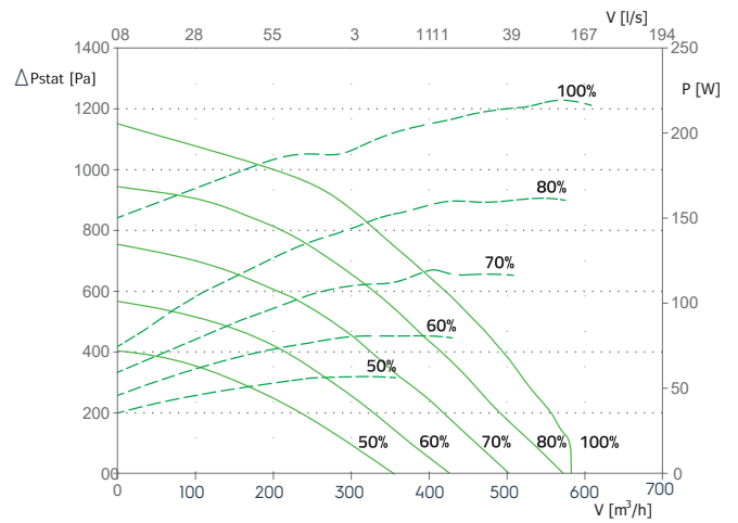
Afvoerlucht
