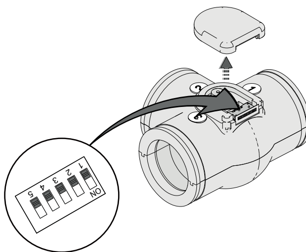
Commutateurs DIP sur le circuit imprimé de la soupape de zone.
