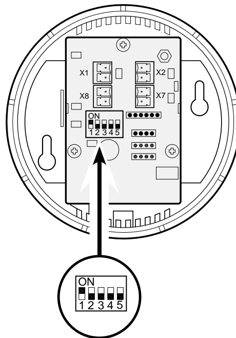
Exemple de réglage de la sonde de CO 2 n°1
