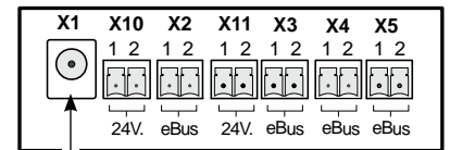
Branchement de l'alimentation 24 V cc
