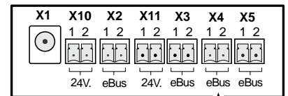
Raccordement eBus vers le récupérateur de chaleur
