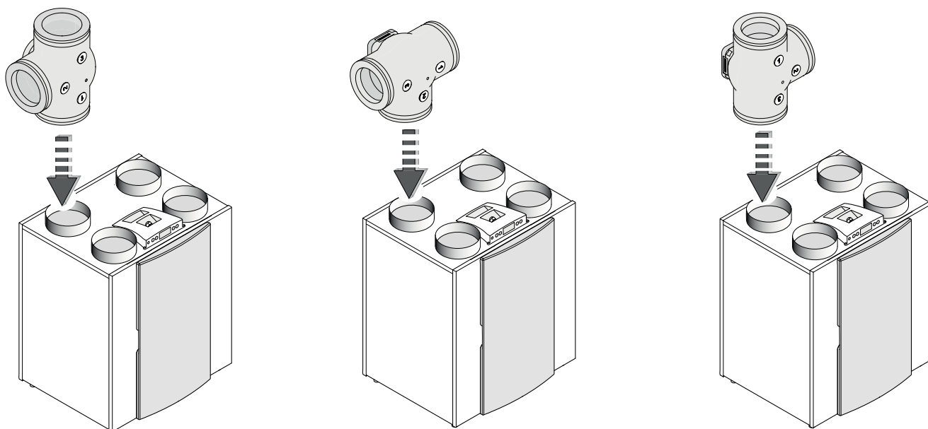
Exemple de raccord d'une soupape de zone sur le conduit d'apport d'air du Renovent Excellent 300 4/0 modèle de droite.
