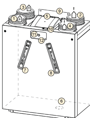
Linker uitvoering
