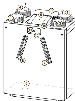
Rechter uitvoering
