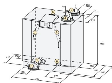
Ubiflux W325 & W400 2/2 gauche
