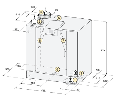
Ubiflux W325 & W400 2/2 droite
