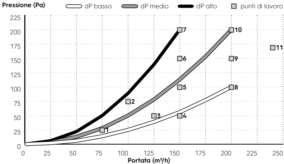
Diagramma portate
